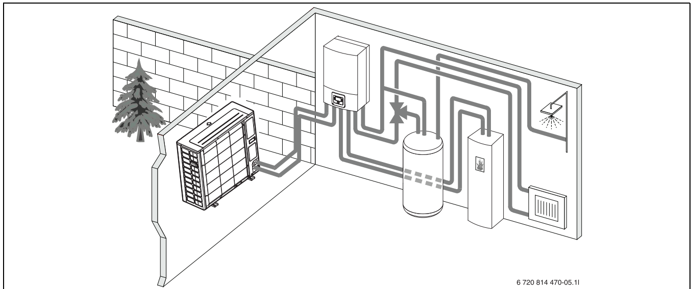
Pav. 2 Išorinio bloko šilumos siurblys, vidinis blokas AWBS be elektrinio kaitintuvo, išorinė karšto vandens talpykla ir išorinis papildomas kaitintuvas
