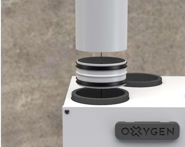
Pav. 3. Oro paėmimo kanalo prijungimo schema
