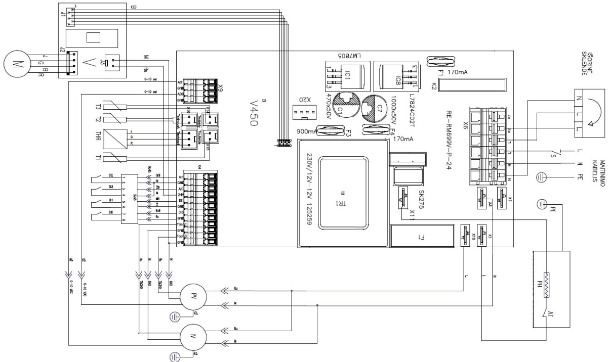
Pav. 9. Vėdinimo įrenginio valdymo plokštės elektrinio jungimo schema
