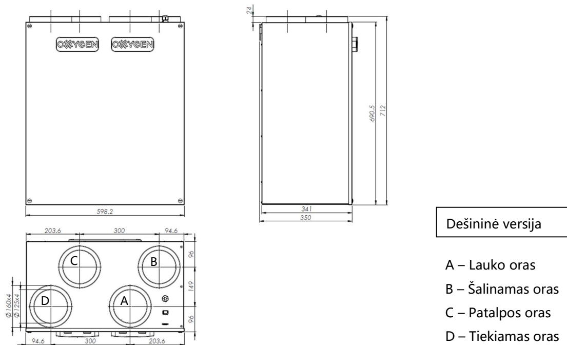
Pav. 1. Vėdinimo įrenginio matmenys
