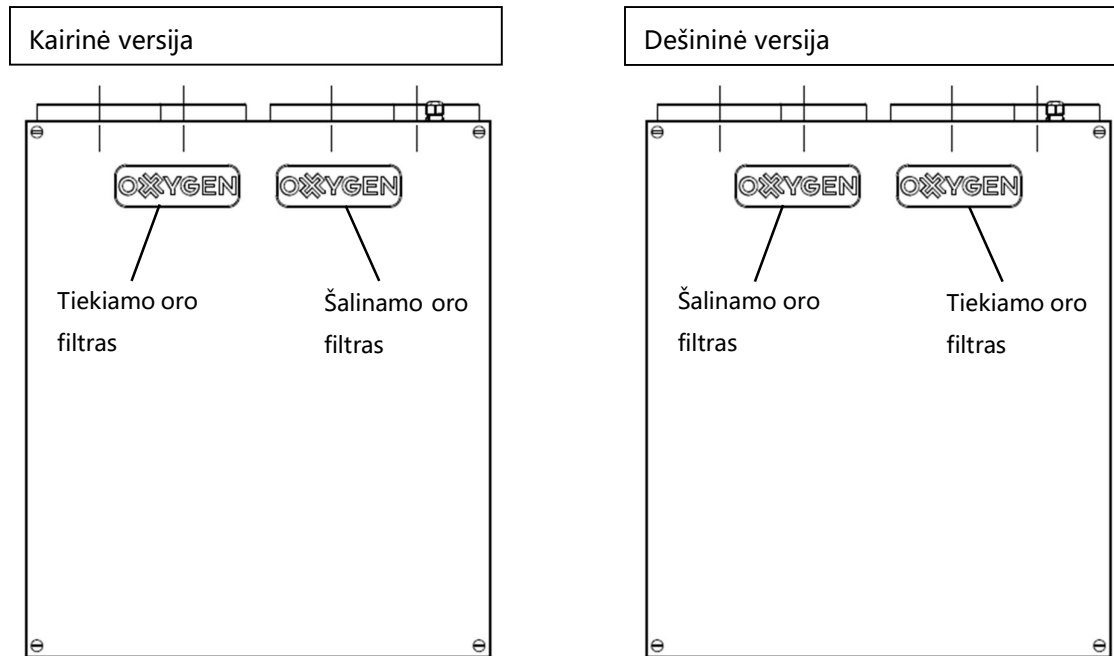
Pav. 10. Vėdinimo įrenginio filtrai
