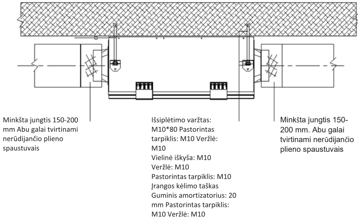
ERV montavimo brėžinys
